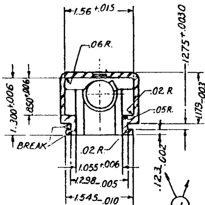
SECTION D-D
