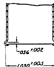
SECTION D-D
